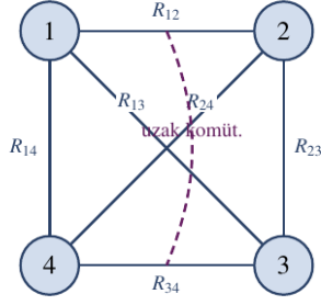
Şekil 9.5 V^{\otimes 4} yerleşimlerinin K_4 grafiği: altı kenar altı R_{ij} , dört üçgen (1,2,3,1,2,4,1,3,4,2,3,4) dört lokal Yang–Baxter kontrolü, ayrık kenar çifti (12)–(34) ise uzak komütativitedir.
