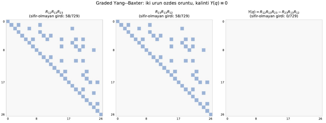
Şekil 9.4 Graded Yang–Baxter denkleminin iki tarafının 27 \times 27 sıfır-olmayan örüntüleri özdeştir; kalıntı Y(q) = R_{12}R_{13}R_{23} - R_{23}R_{13}R_{12} tüm 729 girdide sıfırdır (graded_yang_baxter_residual_GLq21).
