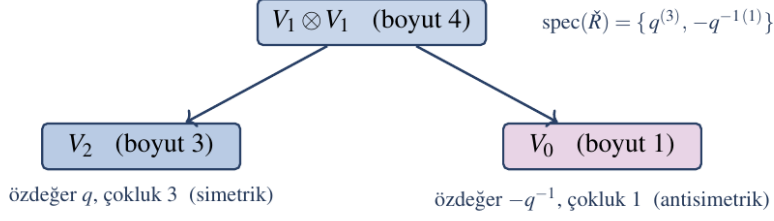
Şekil 8.3 Örgülü \check{R} 'nin spektral ayrışması, V_1 \otimes V_1 = V_2 \oplus V_0 Clebsch–Gordan ayrışımıyla aynıdır. Özdeğer çoklukları doğrudan alt-temsil boyutlarını verir (R_check_eigenvalues).
