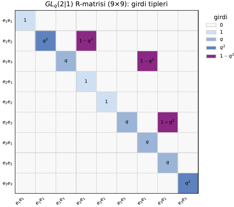
Şekil 9.1 (9.1) R-matrisinin girdi-tipi haritası (R_matrix_GLq21 çıktısı). Köşegen q/q^2 terimleri ile köşegen-dışı 1-q^2 “karışım” terimleri açıkça ayrışır; bu seyreklik, 27 \times 27 ve 81 \times 81 yerleşimlerin neden hâlâ hesaplanabilir kaldığını da açıklar.
