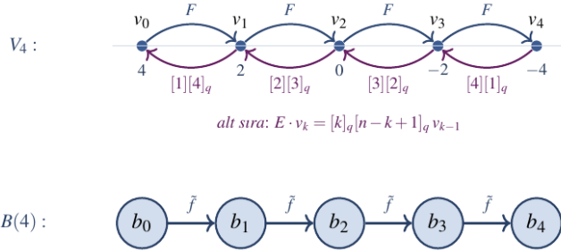
Şekil 4.1 Üstte V_4 temsiliinin ağırlık diyagramı: F (mavi) indeksleri yükseltir, E (mor) q -tamsayı katsayılarıyla geri taşır. Altta aynı temsiliin q \rightarrow 0 kristal gölgesi B(4) , tek tip tilde f oklarıyla.
